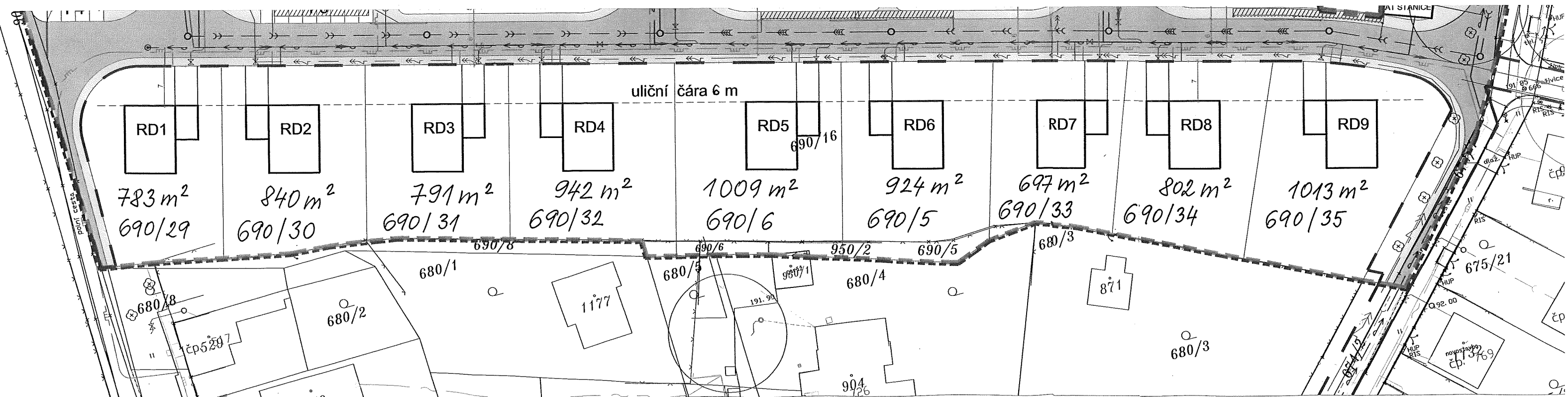
ÚSEK - OBYTNÁ ČTVRŤ "ZA LÁVKAMI" - KOORDINAČNÍ SITUACE 1:500
